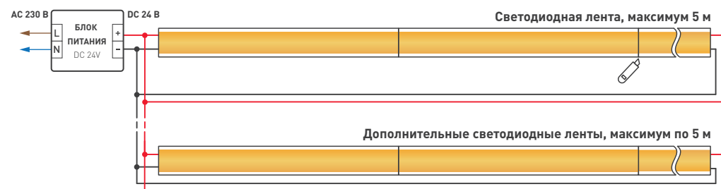
Рис. 1. Подключение нескольких светодиодных лент с двух сторон
