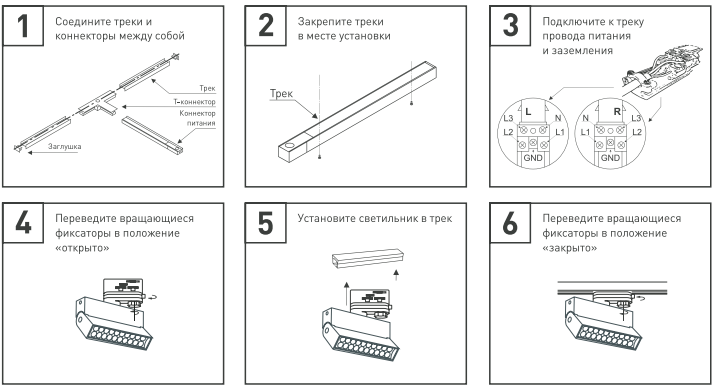
Рис. 2. Установка и подключение светильника
