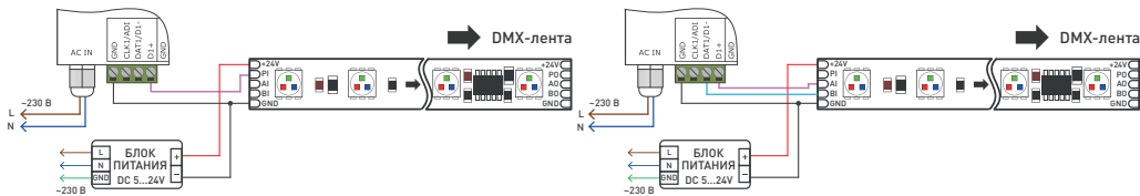
Рисунок 2. Подключение DMX светодиодной ленты к выходу контроллера.
