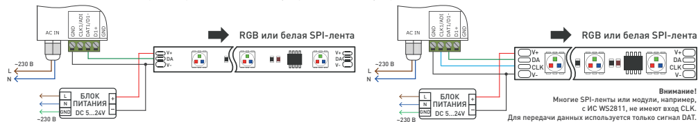
Рисунок 1. Подключение SPI светодиодной ленты к выходу контроллера.
