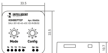
Рис. 1. Габаритный чертеж
