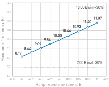
График 1. Зависимость удельной мощности от напряжения питания
