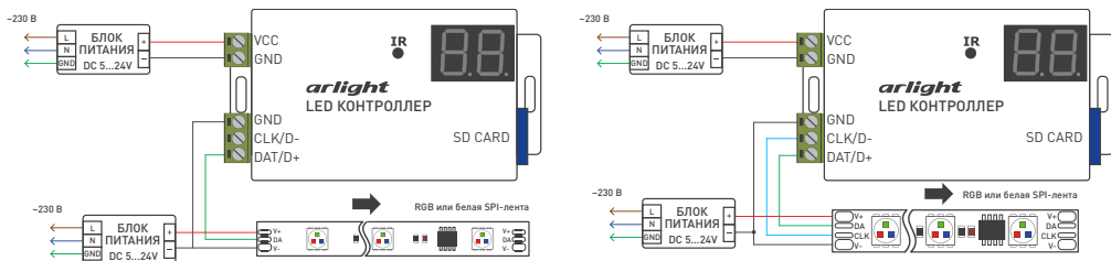
Рис. 1. Подключение SPI-лент к контроллеру
